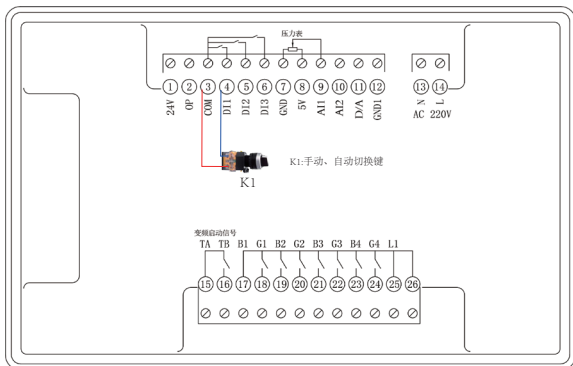
HY920接线端子示意图
